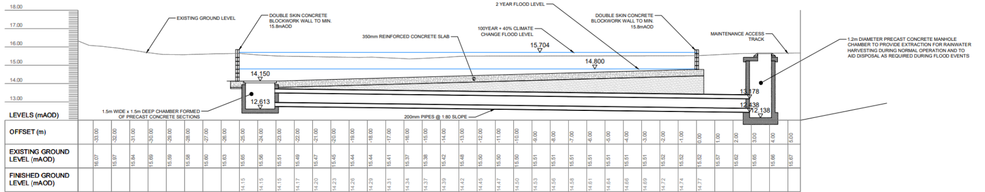
SECTION A-A
